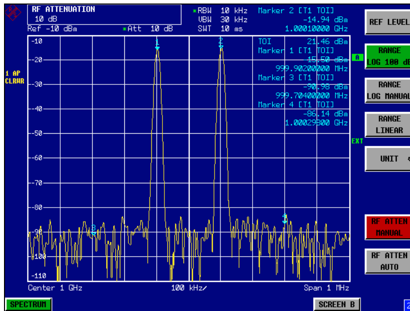
Bild 2-4 Durch Erhöhung der HF-Dämpfung verschwinden die R&S FSP-Eigenstörprodukte im Rauschen.
