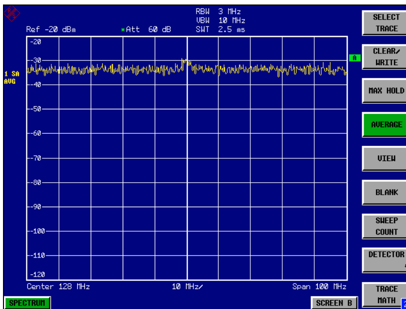
Bild 2-10 Darstellung eines HF-Sinussignals mit geringem Rauschabstand bei Mittelung der Messkurve.
