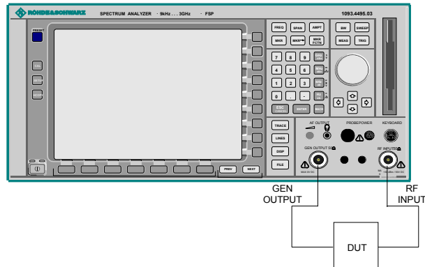
Bild 4-17 Anordnung für Transmissionsmessungen
