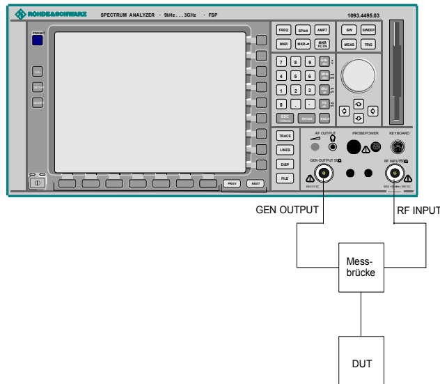
Bild 4-23 Anordnung für Reflexionsmessungen
