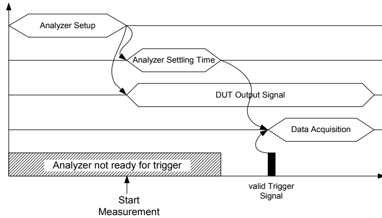
Bild 4-42 Messablauf mit einzelнем Triggerpuls
