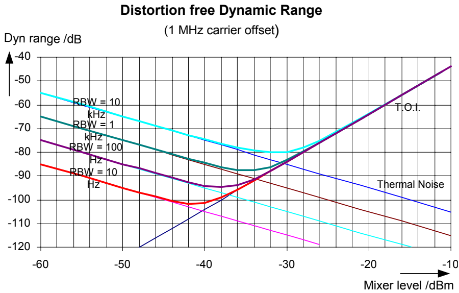
Bild 2-5 Intermodulationsfreier Bereich des R&S FSP3 abhängig vom Pegel am Eingangsmischer und der eingestellten Auflösungsbreite (Nutzsignalabstand = 1 MHz, DANL = -155 dBm / Hz, T.O.I = 12 dBm; typ. Werte bei 2 GHz)
