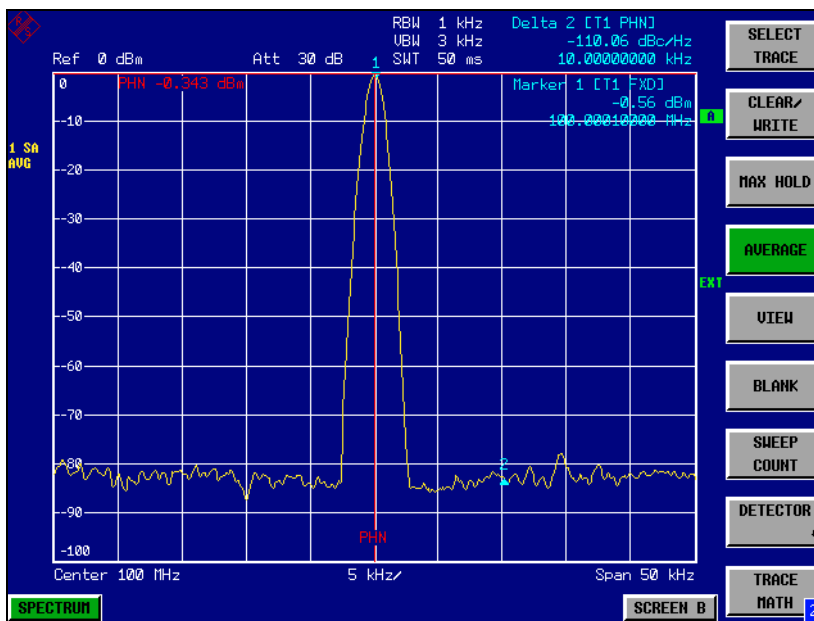
Bild 2-17 Messung des Phasenrauschens mit der Marker-Funktion Phase Noise
