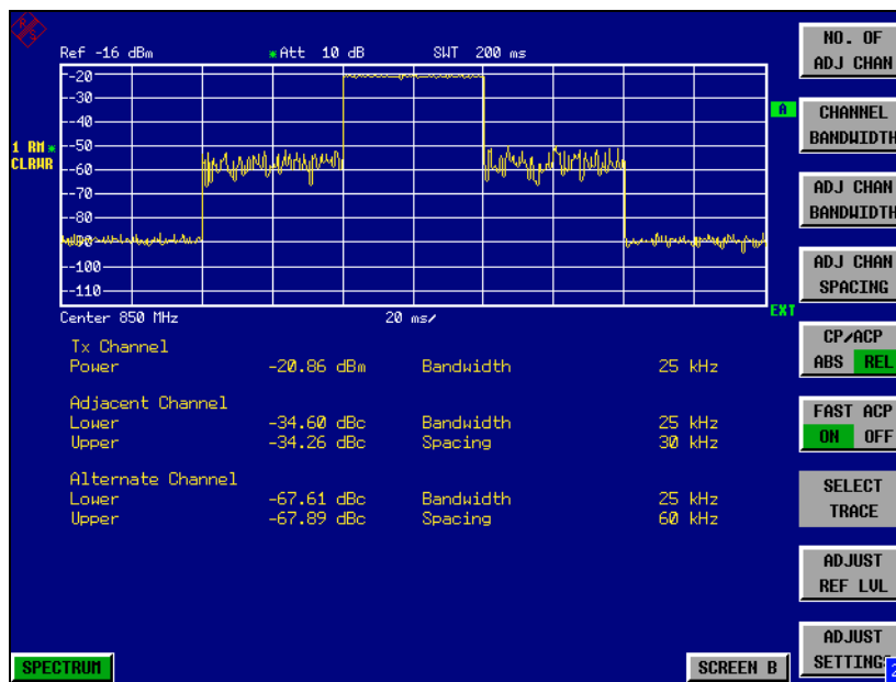
Bild 2-28 Messung der Nachbarkanalleistung im Zeitbereich (Fast ACP)
