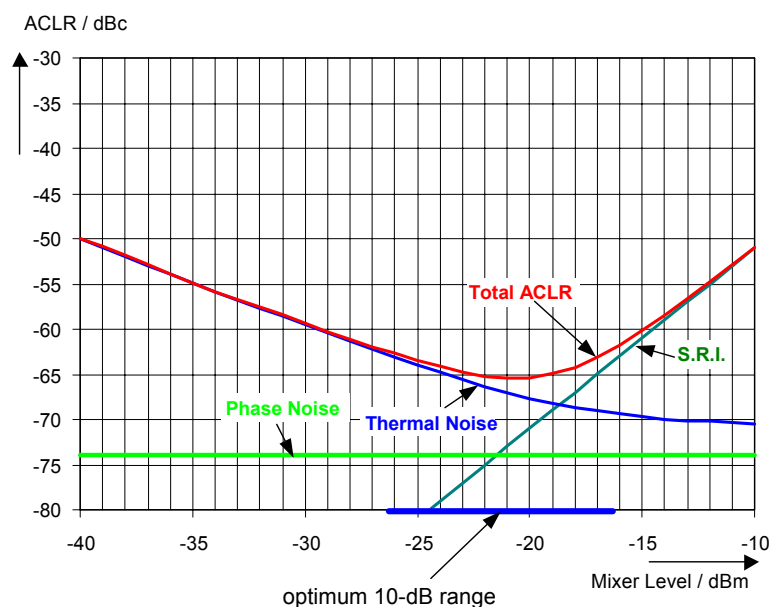
Bild 2-34 Dynamik des R&S FSP bei Nachbarkanalleistungsmessung an W-CDMA-Uplink-Signalen abhängig vom Mischerpegel.
