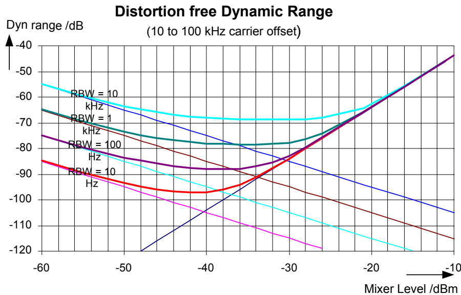
Bild 2-6 Intermodulationsfreier Bereich des R&S FSP3 abhängig vom Pegel am Eingangsmischer und der eingestellten Auflösungsbreite (Nutzsignalabstand = 10 bis 100 kHz, DANL = -155 dBm / Hz, T.O.I = 12 dBm; typ. Werte bei 2 GHz)
