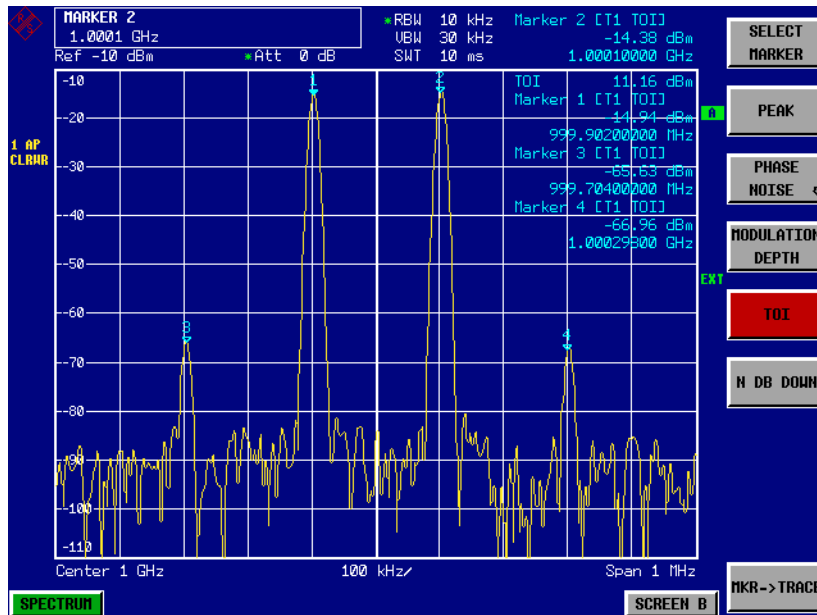
Bild 2-3 Ergebnis der Messung des Eigen-Intermodulationsabstandes des R&S FSP. Der Interceptpunkt dritter Ordnung (TOI) wird am rechten oberen Rand des Grids ausgegeben
