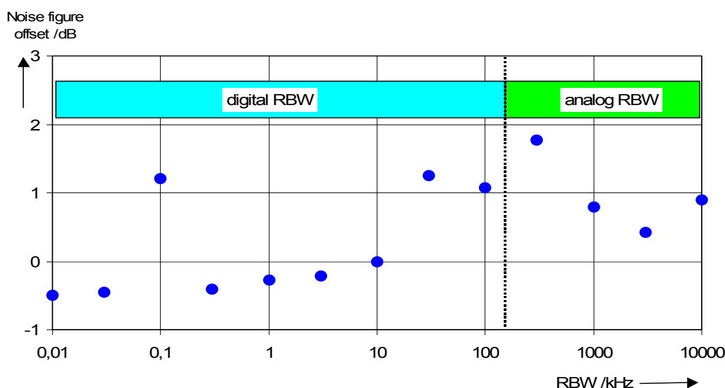
Bild 2-8 Änderung des Rauschmaßes des R&S FSP bei den verschiedenen Bandbreiten. Als Bezugsbandbreite ist 10 kHz gewählt.
