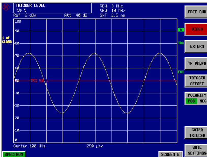
Bild 2-18 Messung des NF-Signals eines mit 1 kHz AM-modulierten Trägers
