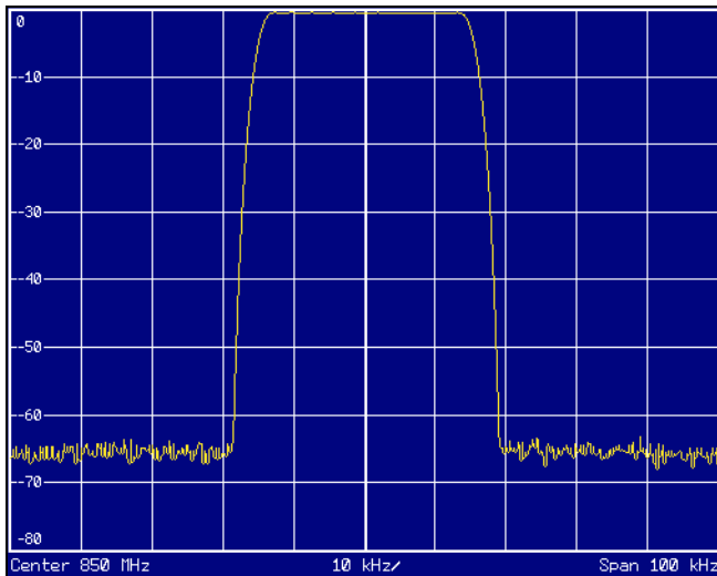
Bild 2-26 Frequenzgang des 30-kHz-Kanalfilters zur Messung der Leistung im IS 95-Nachbarkanal
