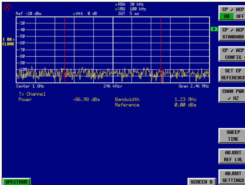
Bild 2-14 Messung der R&S FSP-Eigenrauschleistung in 1,23 MHz Kanalbandbreite.
