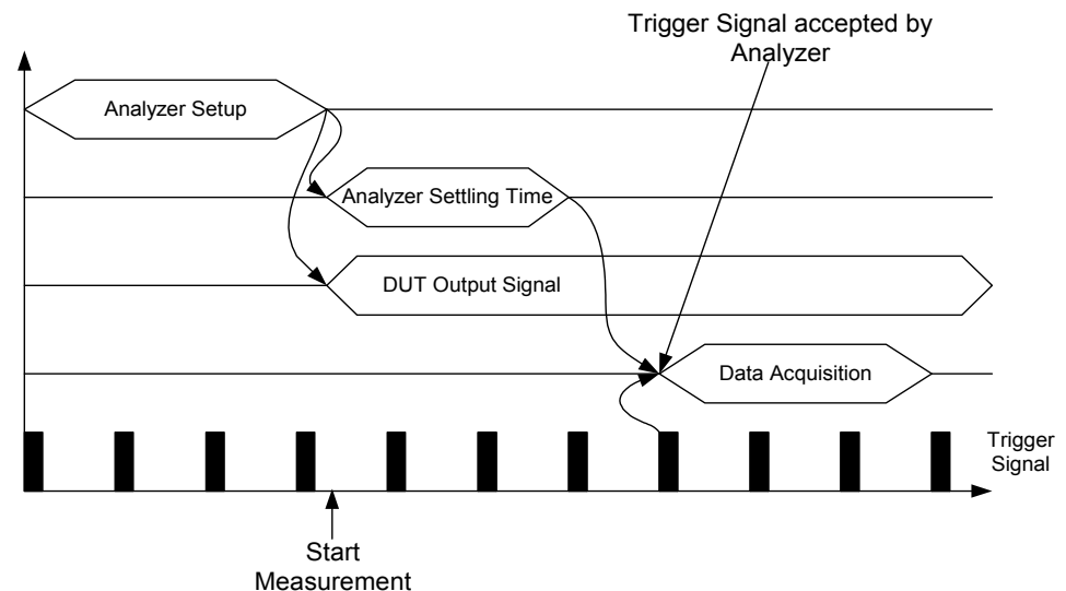
Bild 4-41 Messablauf bei stationärem Messsignal und periodischem Trigger
