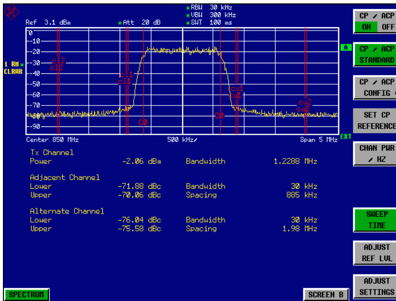
Bild 2-22 Nachbarkanalleistungsmessung an einem CDMA IS95-Signal
