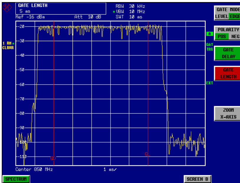
Bild 2-30 Einstellung der Parameter Gate Delay und Gate Length im Zeitbereich. Der Zeitraum, in dem das Spektrum gemessen wird, wird durch zwei senkrechte Linien dargestellt.
