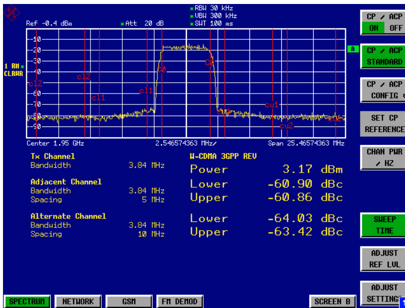
Bild 2-32 Messung der relativen Nachbarkanalleistung an einem W-CDMA-Uplink-Signal.
