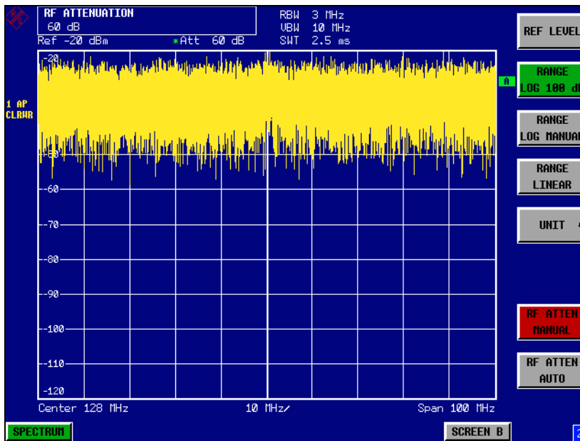
Bild 2-9 Darstellung eines Sinussignals mit kleinem Rauschabstand. Das Signal wird mit dem Auto-Peak-Detektor gemessen fast vollständig durch das Eigenrauschen des Spektrumanalysators überdeckt.
