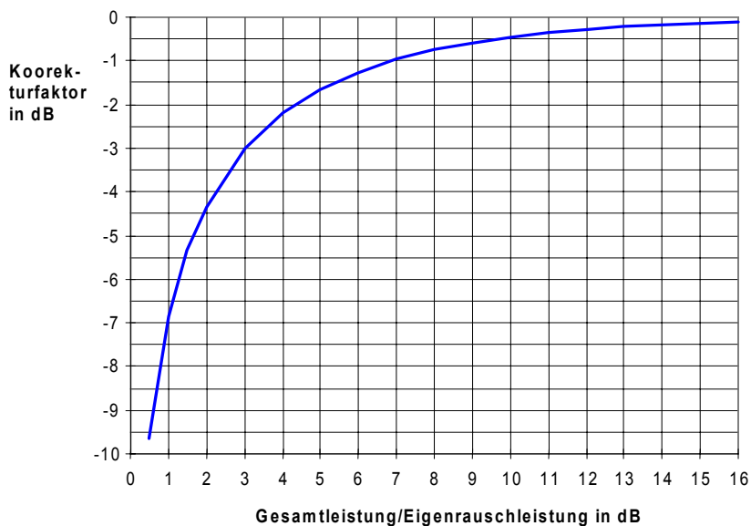
Bild 2-13 Korrekturfaktor für die gemessene Rauschleistung abhängig von Abstand zu Eigenrauschleistung des Spektrumanalysators
