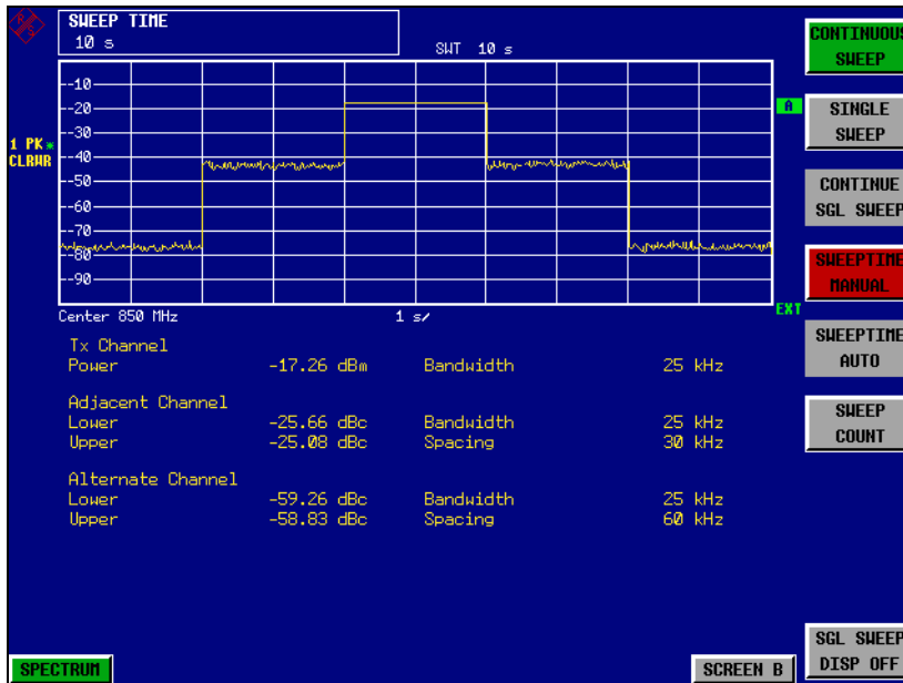
Bild 2-31 Darstellung der Nachbarkanalleistung, die durch das Modulationsspektrum und das Transienzspektrum entsteht
