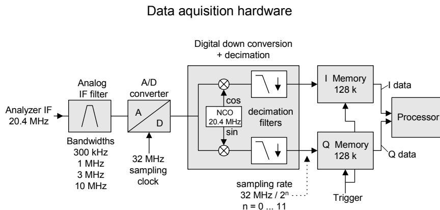
Bild 7-3 Blockschaltbild der Signalverarbeitung des Spektrumanalysator
