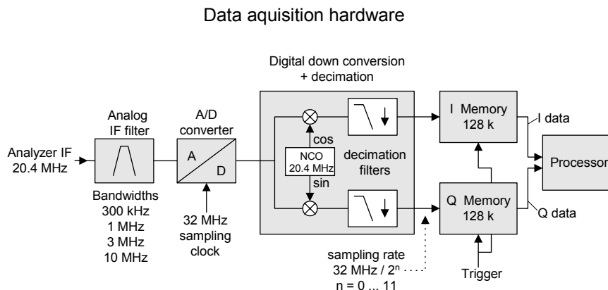
Bild 6-1 Blockschaltbild mit der Signalverarbeitung des R&S FSP
