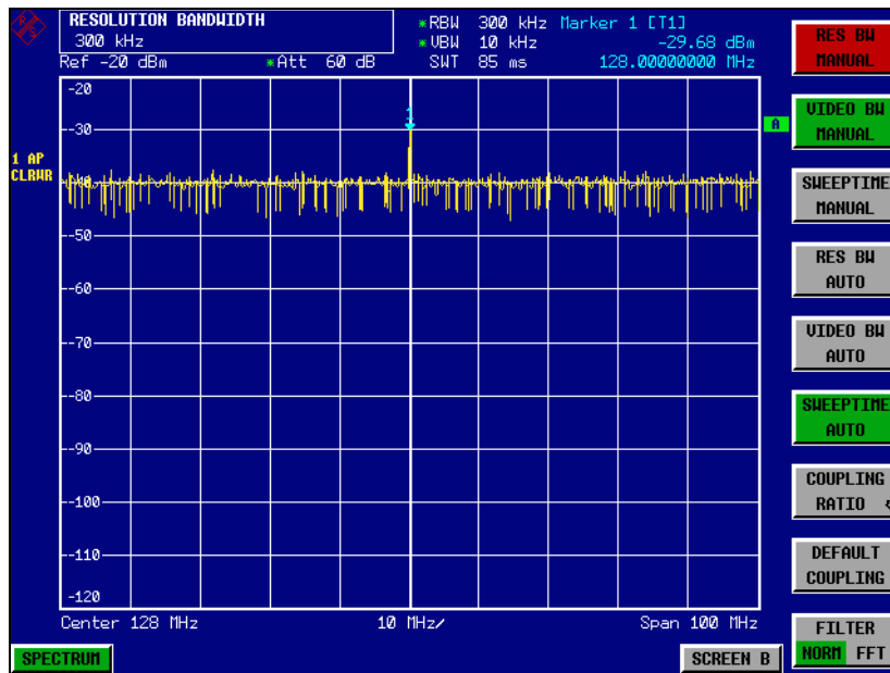
Bild 2-12 Anzeige des Referenzsignals bei kleinerer Auflösebandbreite.
