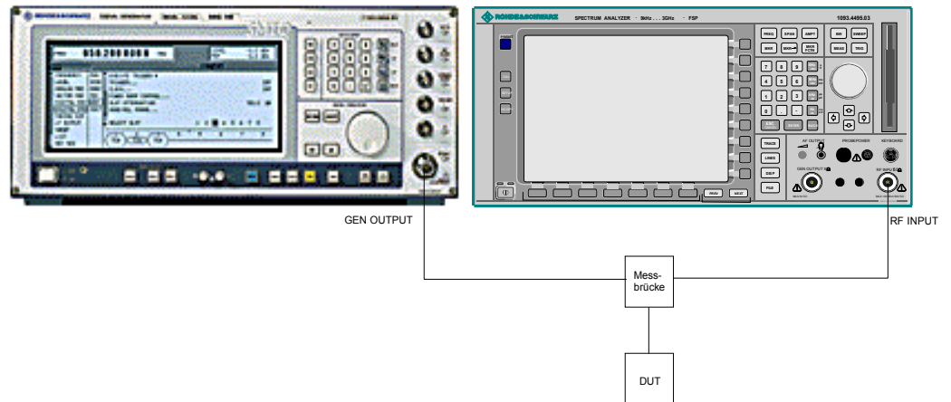
Bild 4-32 Anordnung für Reflexionsmessungen
