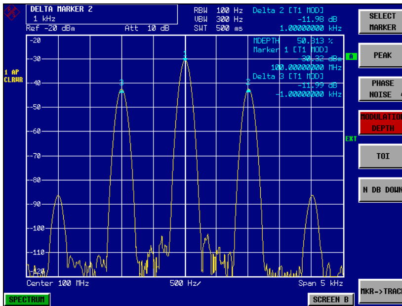
Bild 2-19 Messung des AM-Modulationsgrades. Der Modulationsgrad kann hier mit MDEPTH = 49.436 % abgelesen werden. Die Frequenz des NF-Signals kann der Frequenzanzeige der Delta-Marker entnommen werden
